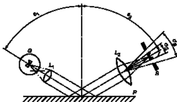
G — лампа; L 1 , L 2 — линзы; В — полевая диафрагма приемного устройства; P — лакокрасочное покрытие; ε 1 — угол падения, ε 2 — угол отражения (ε 1 = ε 2 ); α B — апертурный угол приемной системы; α G — апертурный угол изображения источника, I — изображение нити накала
